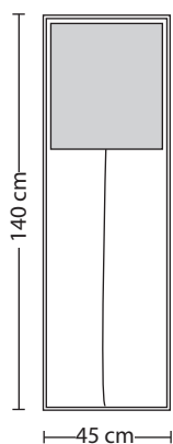
Namibië floorlamp front view
